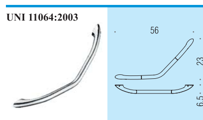
B9735 Maniglione da vasca Bath grab-bar
