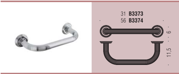
B3373 - B3374 Maniglione da vasca Bath grab-bar
