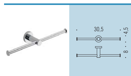
W4990 Porta rotolo doppio Double Paper holder
