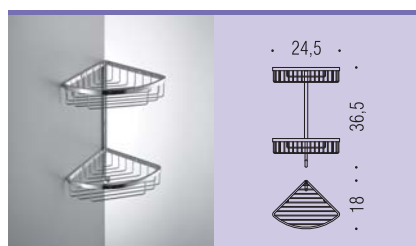
B9617 Angolare doppio con gancio Double corner basket with hook
