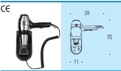
B9994 VAMA Asciugacapelli da parete con presa universale per rasoio 110/220V Automatic wall hair dryer with universal shaver socket 110/220V
