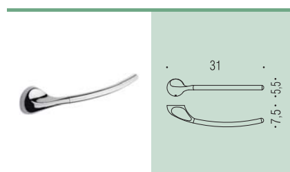
B1211 Porta salvietta fisso Towel holder
