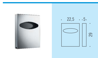
B9972 Distributore copri-water monoblocco (200 pz.) con serratura di sicurezza - acciaio inox WC seat covers (200 pcs) dispenser, with security lock
