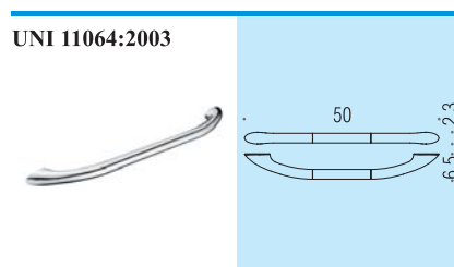
B9734 Maniglione da vasca Bath grab-bar
