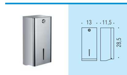
B9976 Distributore di salviette di carta con serratura di sicurezza - acciaio inox Stainless steel tissue dispenser with safety lock
