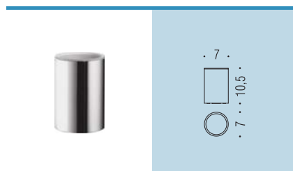
W4941 Porta bicchiere d'appoggio Standing glass holder
