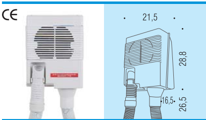
B9973 VAMA Asciugacapelli da parete con tubo flessibile Wall mounted hair dryer with flexible tube
