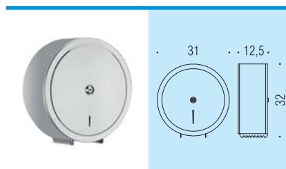
B9983N Distributore rotoli carta igienica con serratura di sicurezza - acciaio inox Stainless steel rollpaper dispenser with safety lock
