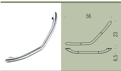
B9735 Maniglione da vasca Bath grab-bar conforme - it complies with UNI 11064:2003
