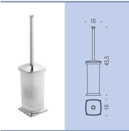
B3206 Porta scopino d'appoggio Standing brush holder
