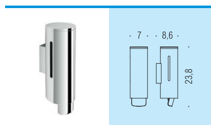
B9979N Spandisapone (L 0,35) Soap dispenser
