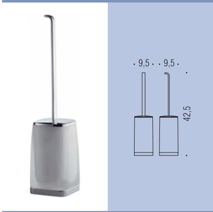
W4206 Porta scopino d'appoggio Standing brush holder
