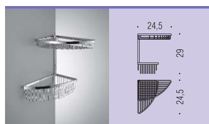
B9609 Angolare doppio Double corner basket
