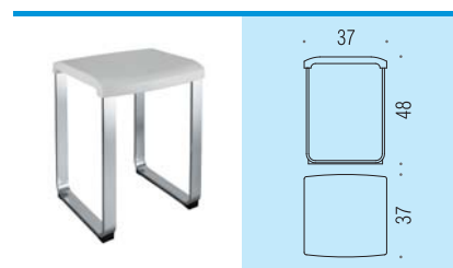
B9967 FLAT Sgabello. Seduta: in resina termoplastica. Struttura: in alluminio anodizzato FLAT Seat. Seat: thermoplastic resin. Frame: anodized aluminium
