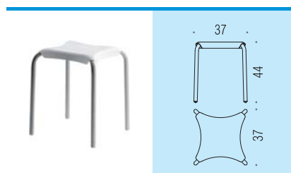
B9955 SIT Sgabello. Seduta: in ABS bianco. Struttura: in alluminio verniciato con polvere epossidica grigia SIT Seat. Seat: white ABS. Frame: grey epoxy powder coated aluminium
