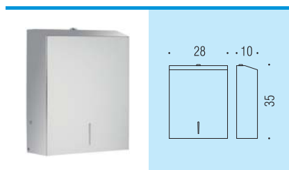
B9960N Distributore di salviette di carta con serratura di sicurezza - acciaio inox Stainless steel tissue dispenser with safety lock
