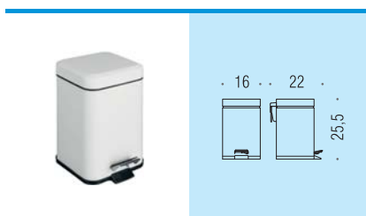
B9210 Poubelle in acciaio inox verniciato (L 3) con sistema di chiusura ammortizzata Small pedal bin, varnished stainless steel with amortized closure
