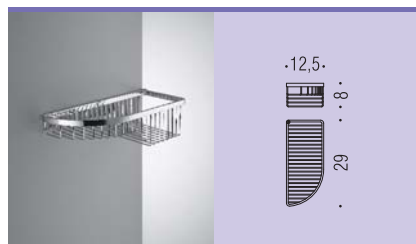
B9608 Angolare semplice Single corner basket
