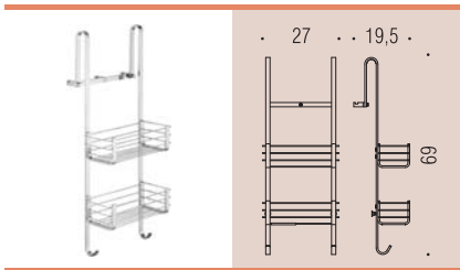
B9634 “Cavalletto” porta oggetti universale per box doccia Universal rack for shower-box
