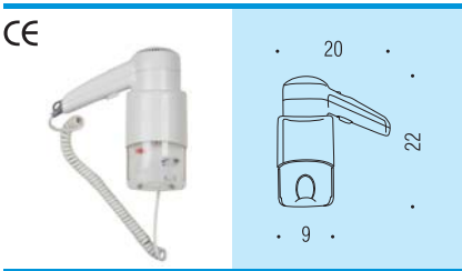
B9995 VAMA Asciugacapelli da parete con presa universale per rasoio 110/220V Automatic wall hair dryer with universal shaver socket 110/220V
