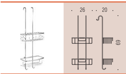
B9635 “Cavalletto” porta oggetti universale per box doccia Universal rack for shower-box
