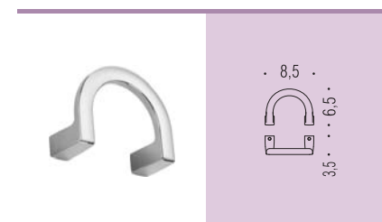
LC47 Appenditutto Hook
