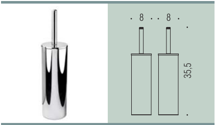
B2706 Porta scopino d'appoggio Standing brush holder
