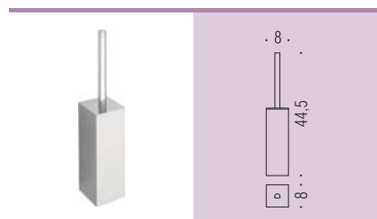
B6206 Porta scopino d'appoggio Standing brush holder
