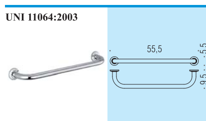
B9721 Maniglione da vasca Bath grab-bar
