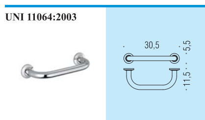
B9720 Maniglione da vasca Bath grab-bar
