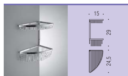
B9612 Angolare doppio Double corner basket
