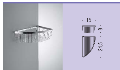
B9610 Angolare semplice Single corner basket
