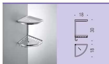
B9601 Angolare doppio con cestino, vaschetta in ceramica e gancio Double corner basket with ceramic bowl and hook
