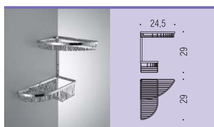
B9607 Angolare doppio Double corner basket
