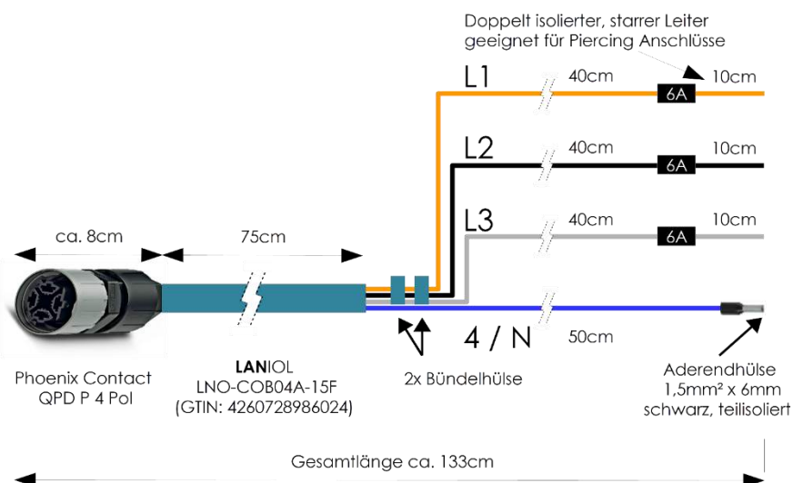
LNO-EXTBPL-01 16 - 120mm²
